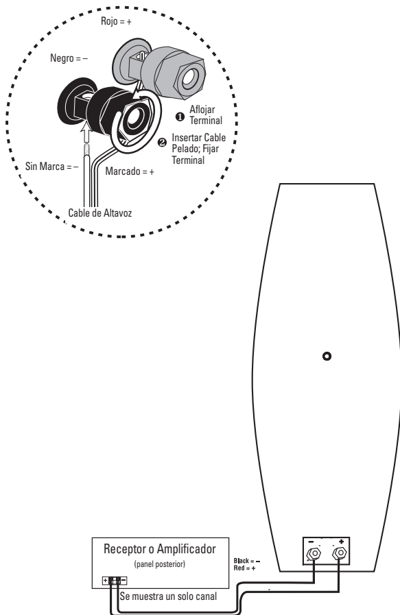
Figura 3. El diagrama de cableado muestra la polaridad de las conexiones de un canal de sistema de cine doméstico.
